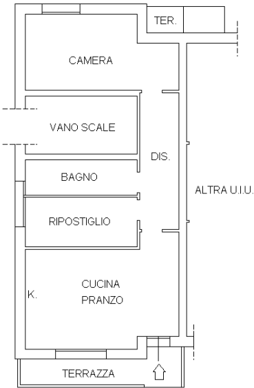
PIANTA PIANO TERRA H: 270
